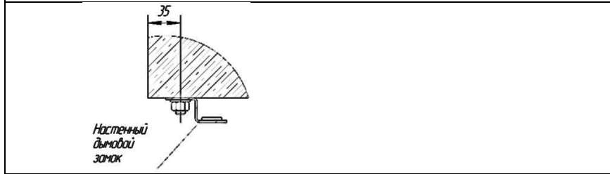
9. Установка настенного дымового замка
