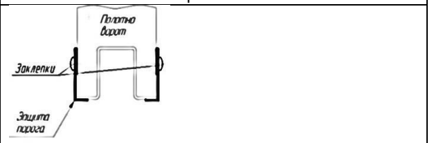
16. Установка защиты порога
