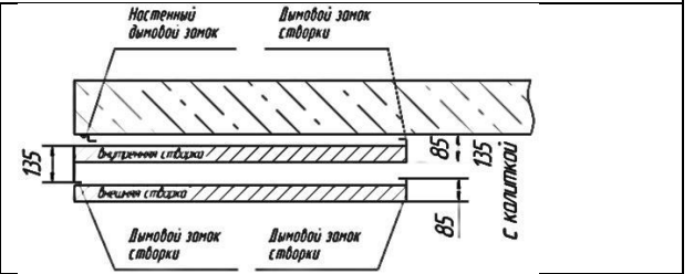
10. Установка на створки дымовых замков
