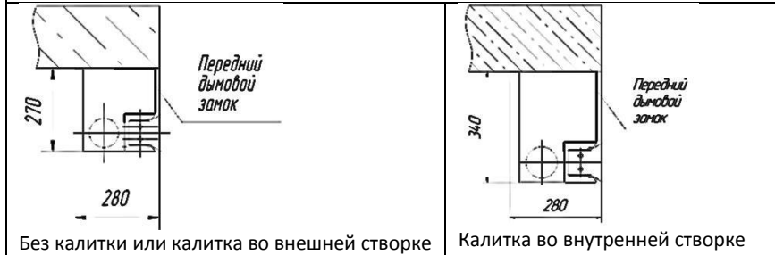
17. Установка переднего дымового замка
