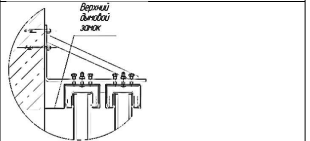
18. Установка верхнего дымового замка (если калитка во внутренней створке)
