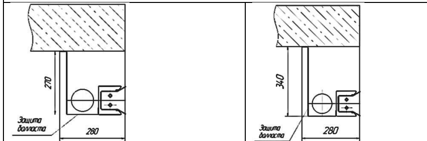
13. Монтаж защиты балласта
