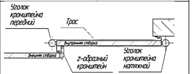
12. Схема соединения створок тросом (кронштейны установить наверху створок)
