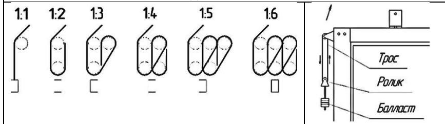
11. Установка балласта
